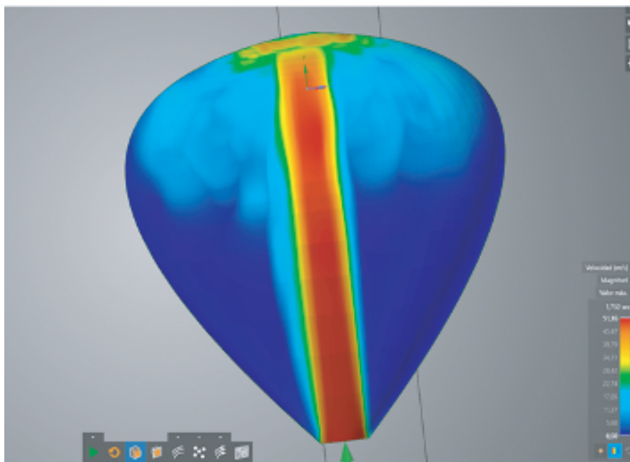
Figura 6. Simulación fluida interno Discovery Live 2020 R1 ®. Escala 1:1
