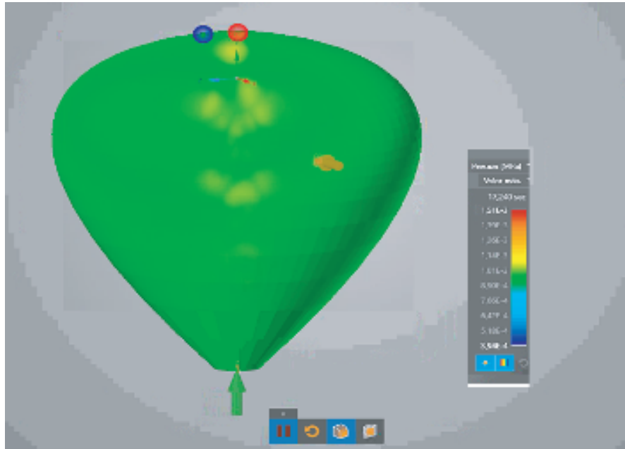
Figura 7. Simulación presión interna Discovery Live 2020 R1 ®. Escala 1:1
