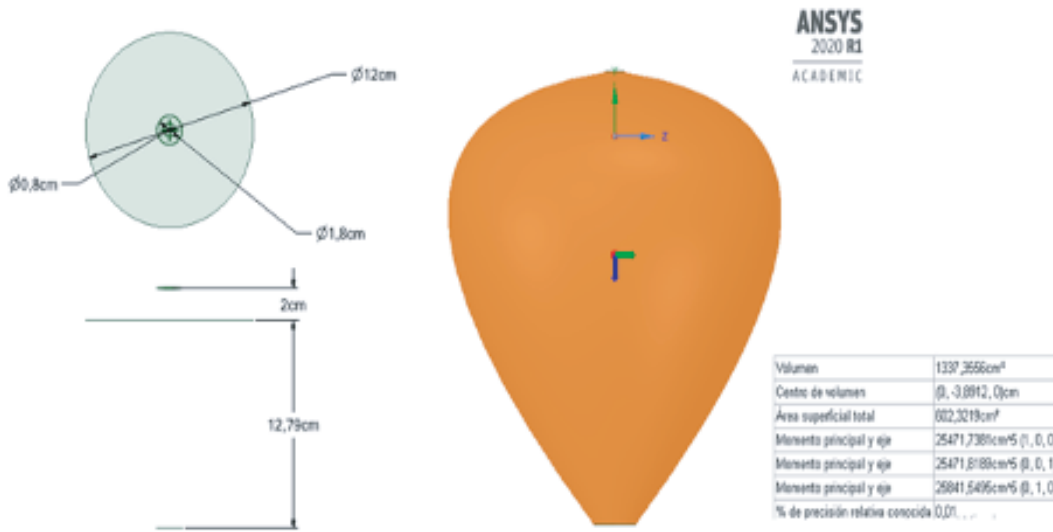
Figura 4. Diseño en Ansys Space Claim 2020 R1 ® Academic. Escala 1:100
