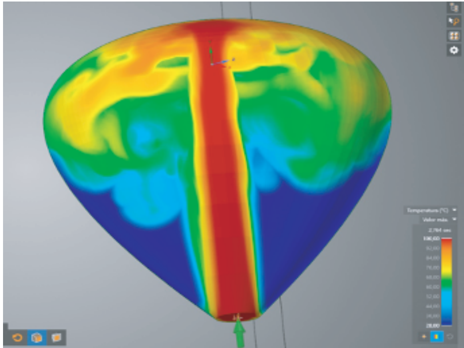
Figura 5. Simulación térmica Discovery Live 2020 R1 ®. Escala 1:1
